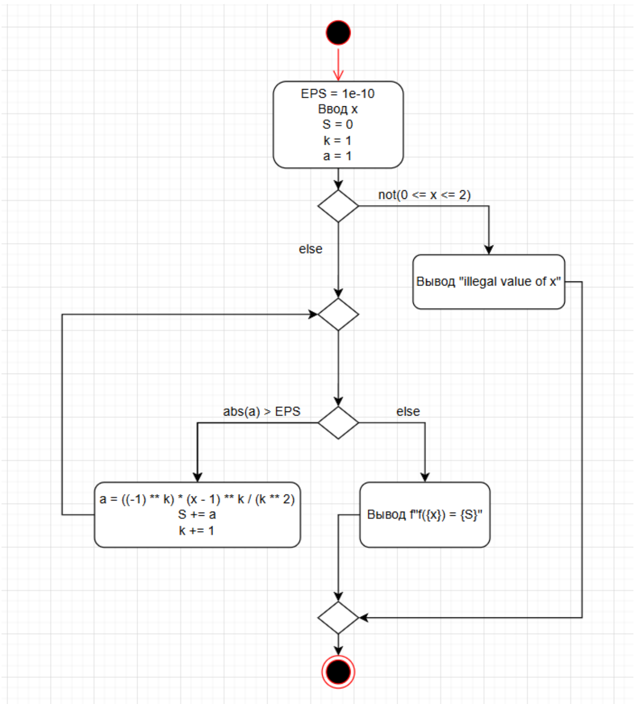
Рисунок 24. UML-диаграмма решения задания повышенной сложности
